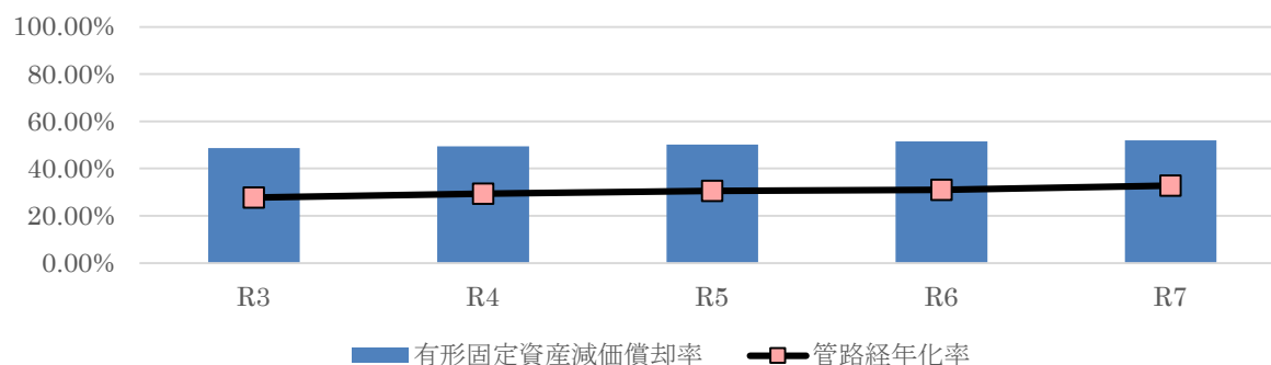
有形固定資産減価償却率・管路経年化率の推移
