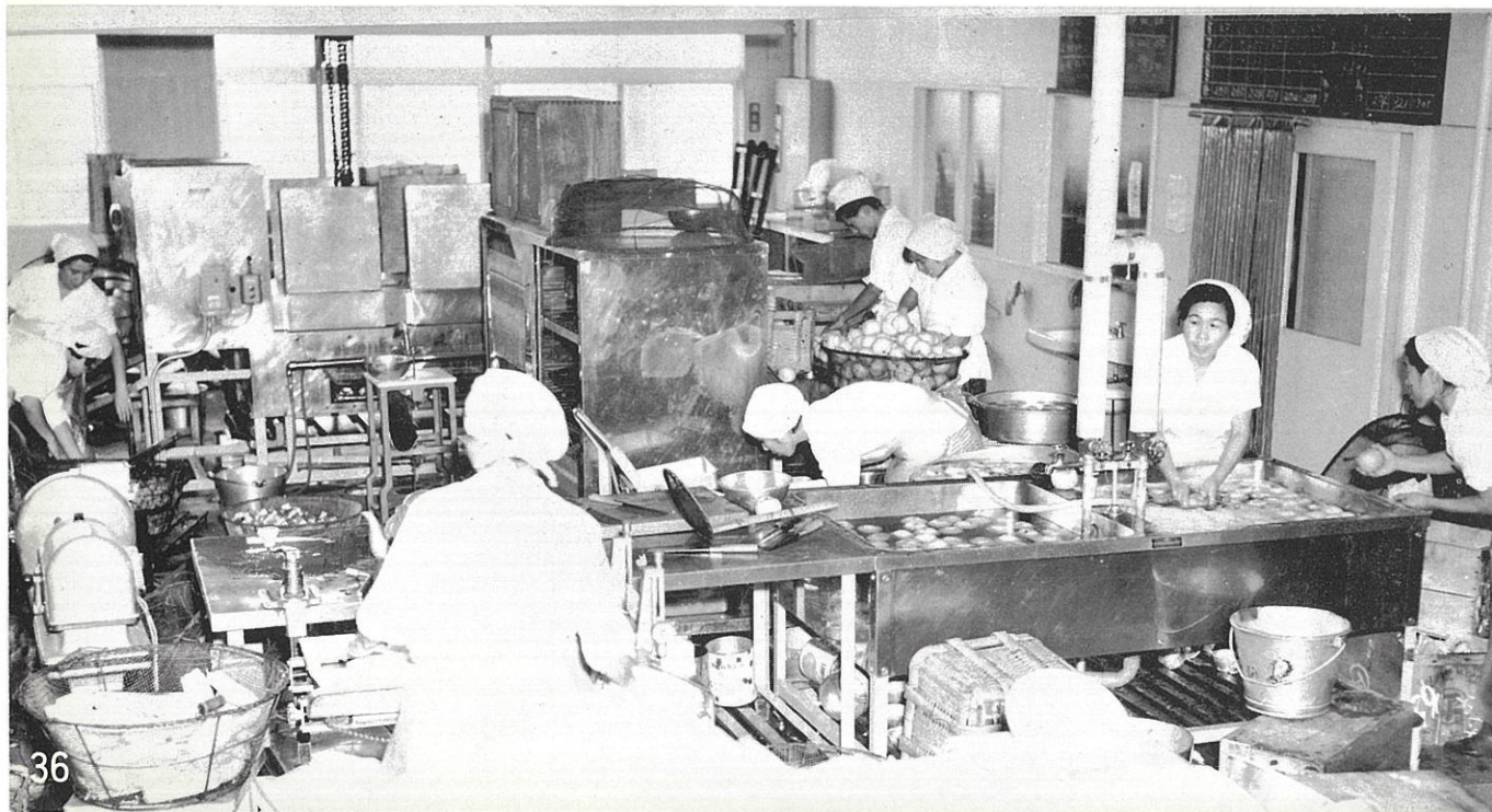
給食センター調理室
