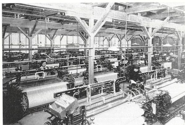
瀧田繊維工場織布部(西浦町)
