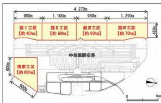
▲中部国際空港沖公有水面埋立事業
