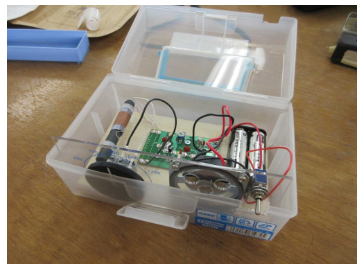
※常滑アマチュア無線クラブ オリジナルのキットで制作
