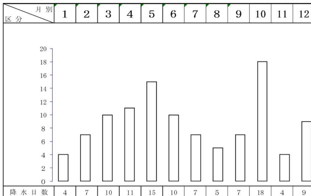
月別降水日数・降水量
